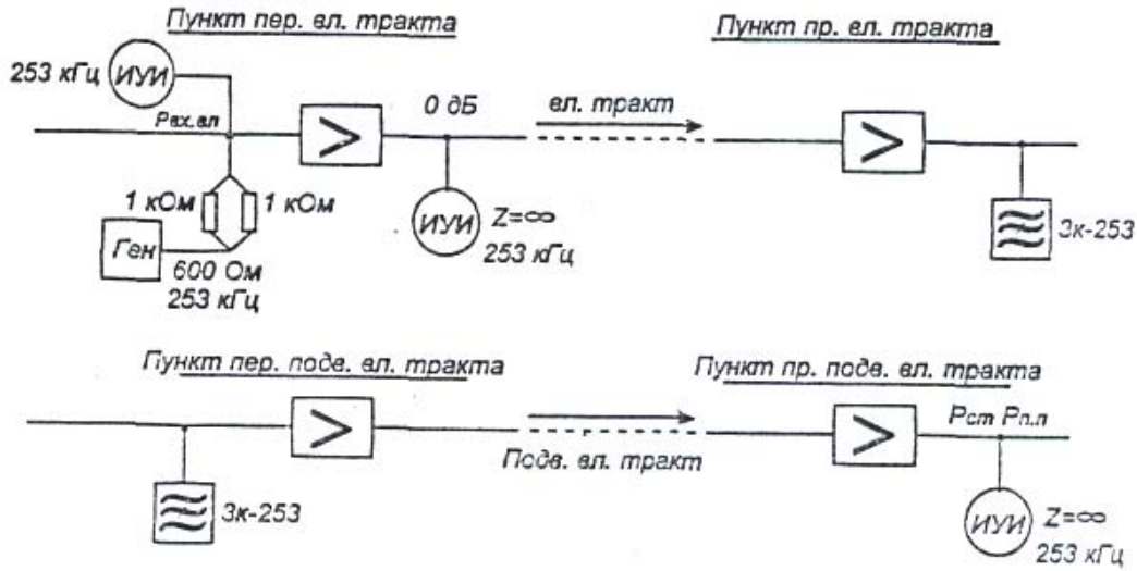
Рис. 1. Измерение защищенности на дальнем конце
