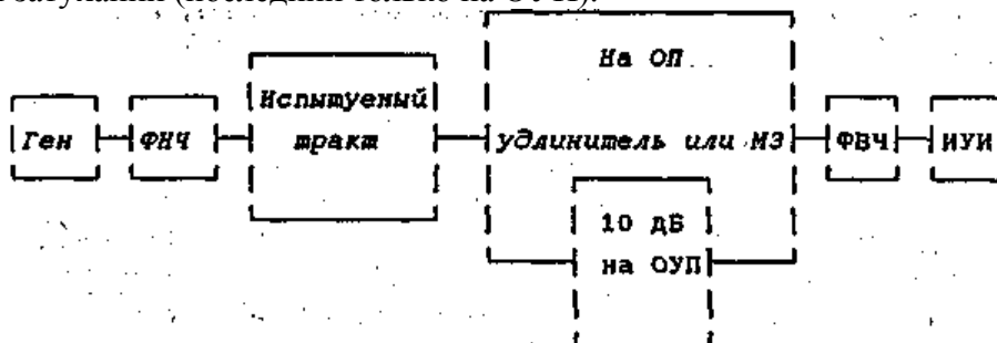
Схема измерений
