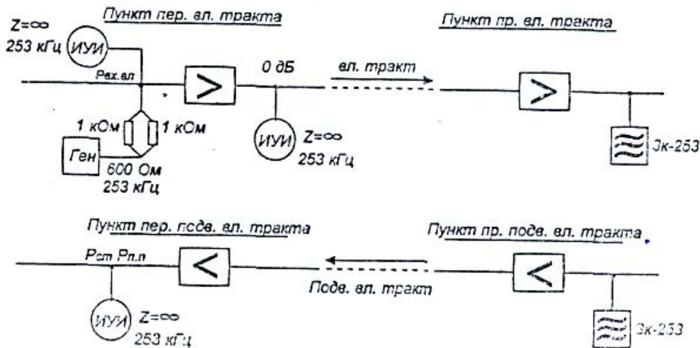
Рис. 2. Измерение защищенности на ближнем конце
