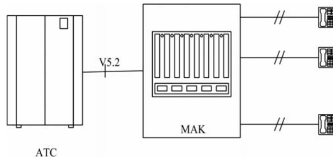
Рис. 1.1. Включение аналоговых абонентских линий в концентратор с V5
