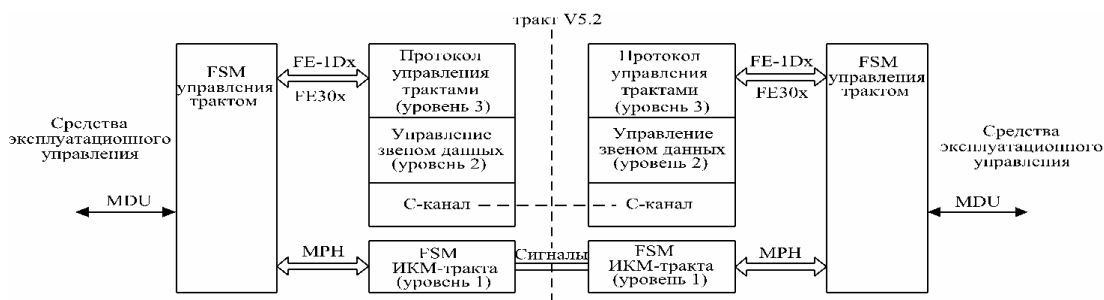
Рис. 7.1. Функциональная модель управления трактом интерфейса V5.2
