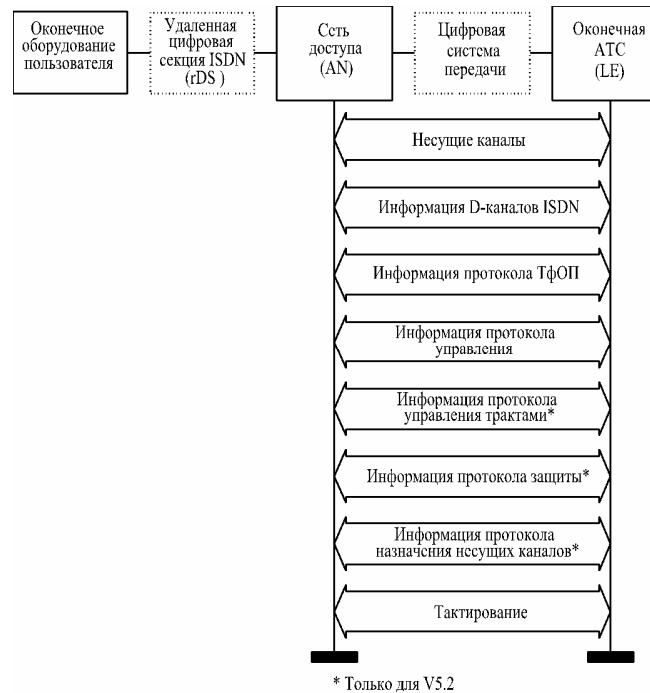
Рис. 1.5. Функциональная модель доступа через интерфейс V5.2
