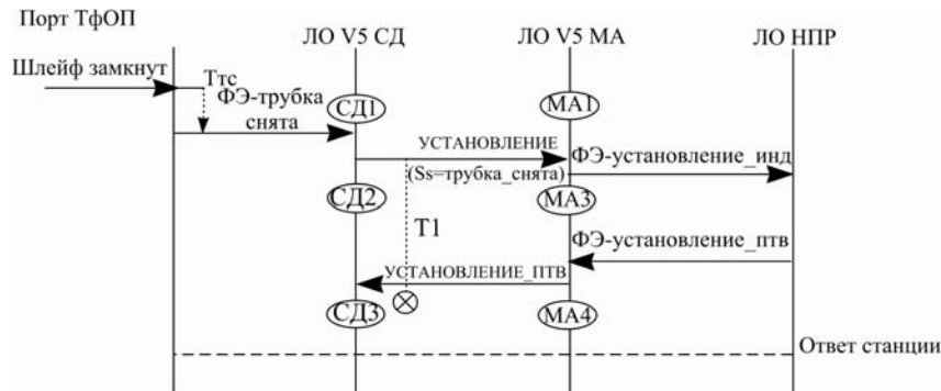
Рис. 5.4. Передача сообщений и сигналов FE: исходящий вызов
