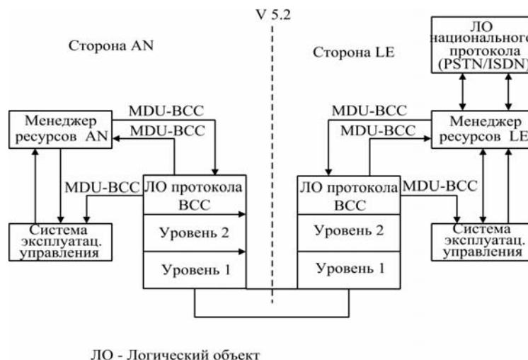
Рис. 8.1. Функциональная модель интерфейса протокола ВСС
