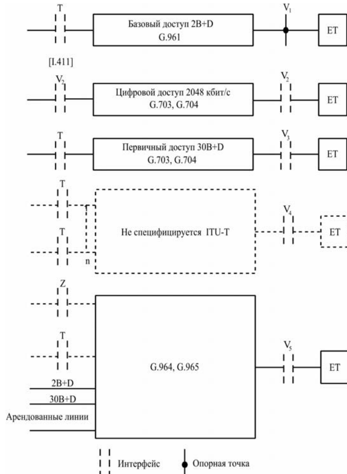
Рис. 1.4. Возможные варианты доступа в точке V
