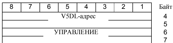
Рис. 2.3. Структура А-кадра (без информационного поля)
