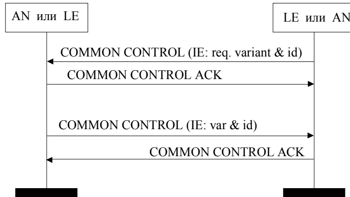
Рис. 10.4. Процедура идентификации тракта
