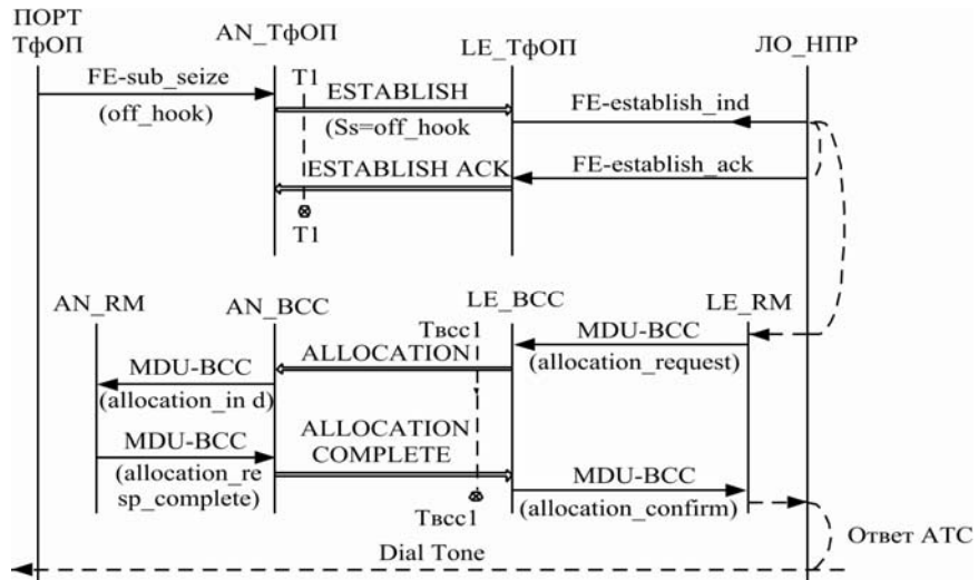
Рис. 8.2. Исходящий вызов. Нормальная процедура
