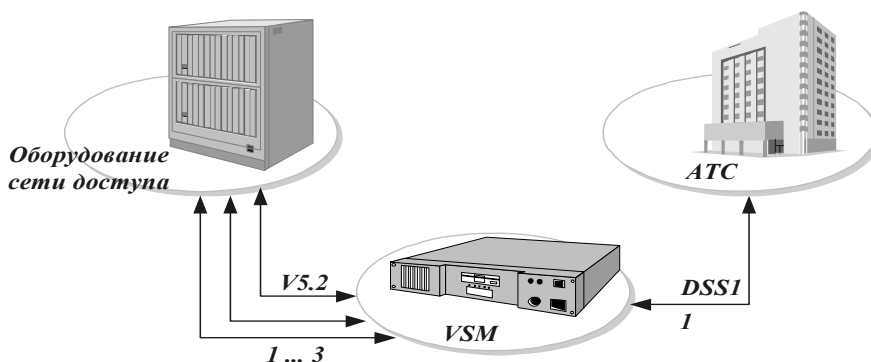
Рис. 11.3. Включение конвертера
