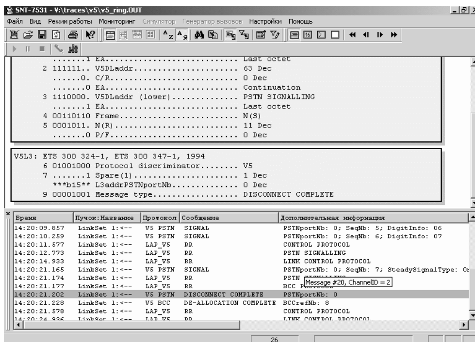
Рис. 10.6. Окно режима мониторинга
