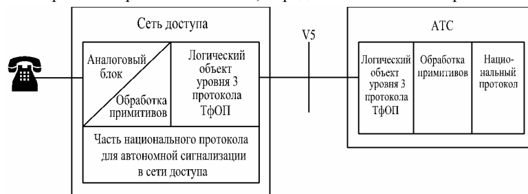
Рис. 3.1. Функциональная модель пользовательского порта ТфОП
