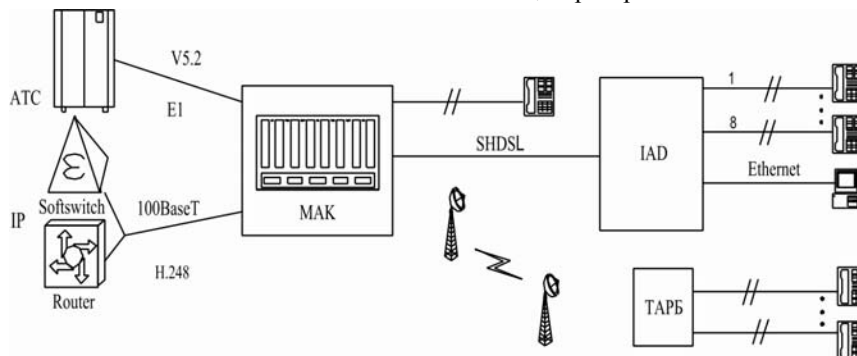
Рис. 1.3. Универсальный вариант включения MAK
