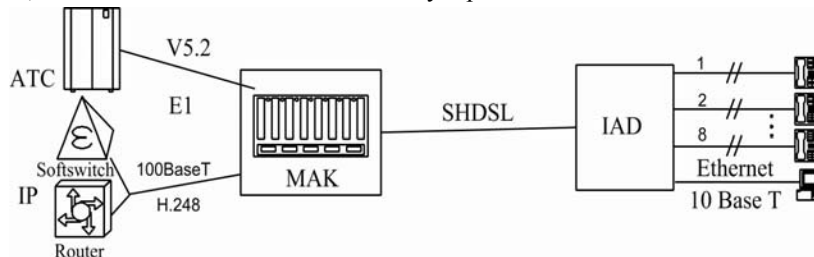
Рис. 1.2. Включение IAD в концентратор с V5
