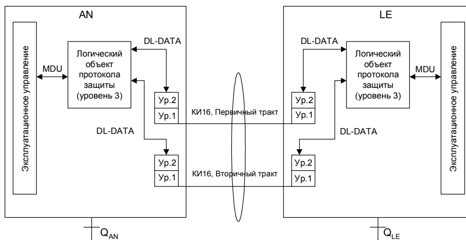
Рис. 9.2. Функциональная модель протокола защиты
