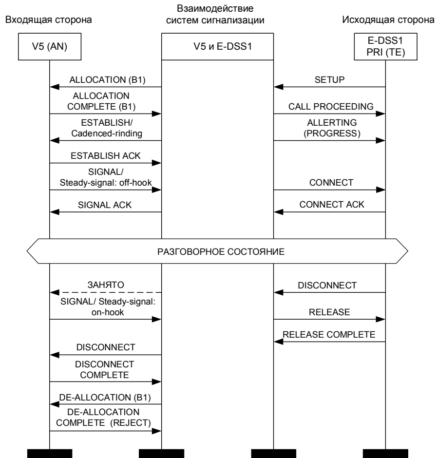
Рис. 11.1. Вызов к свободному абоненту. Отбой абонента А
