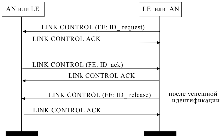
Рис. 10.3. Проверка : «Variant» и «Interface_ID»
