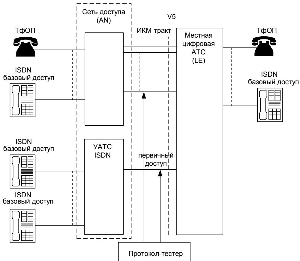
Рис. 10.1. Тестируемая конфигурация
