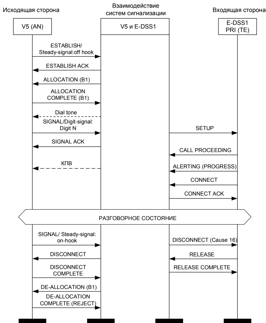
Рис. 11.2. Вызов к свободному абоненту. Декадный код. Отбой абонента А
